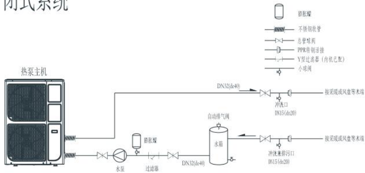
图4.2水循环系统安装示意图
